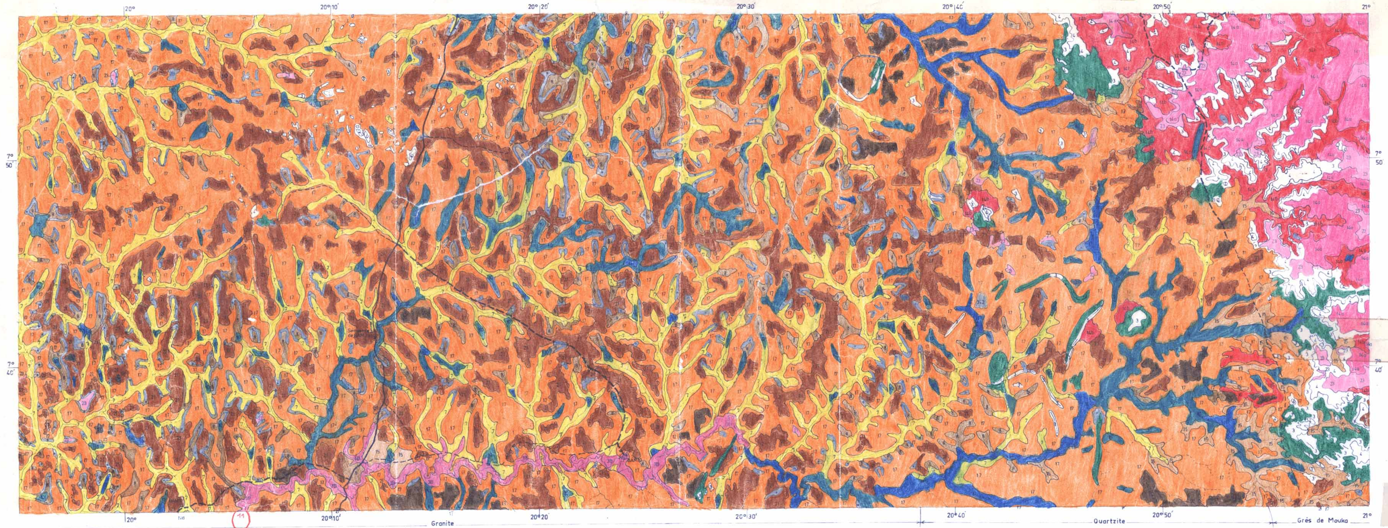
LÉGENDE DE L'ESQUISSE PEDO-GEOMORPHOLOGIQUE DES ENVIRONS DE BAMINGUI
