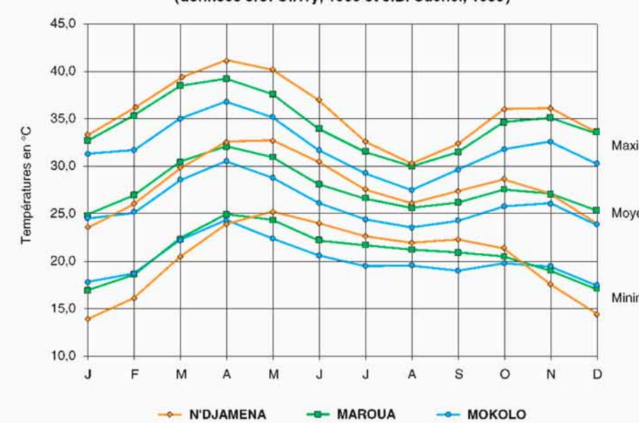
Carton 7 - Températures moyennes mensuelles maximales, moyennes et minimales (données J.C. Olivry, 1986 et J.B. Suchel, 1988)
