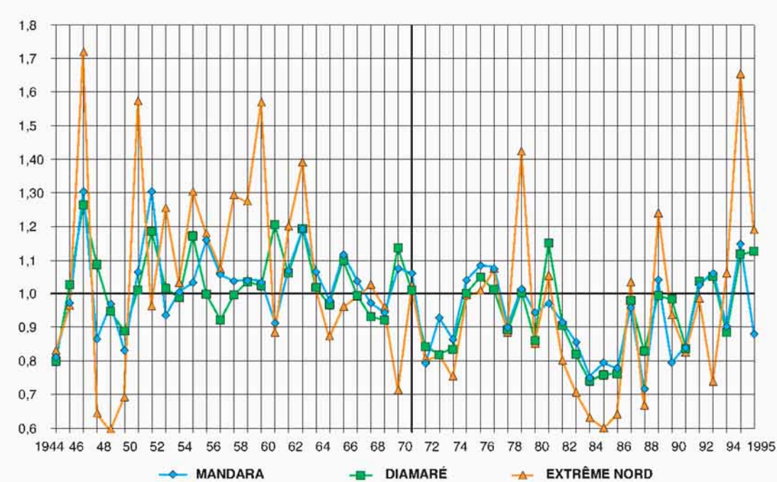
Carton 4 - Vecteurs pluviométriques annuels régionaux (période 1944-1995)
