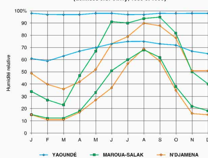
Carton 8 - Moyennes mensuelles des humidités relatives maximales et minimales (données J.C. Olivry, 1986 et 1996)
