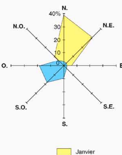
Carton 6 - Rose des vents en janvier et août à Maroua-Salak : pourcentages des directions moyennes observées (période 1961-1970)
